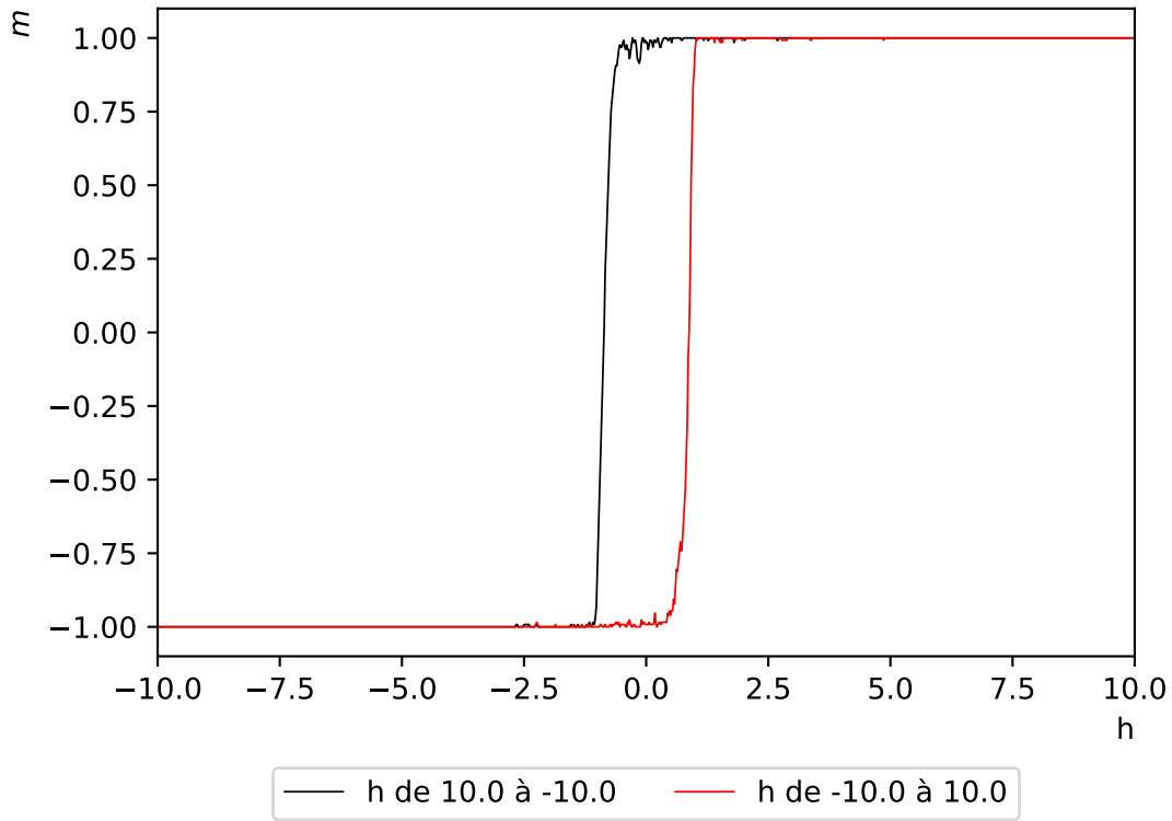
Hystérésis de l'aimantation - réseau de taille L=16 - champ magnétique d'amplitude h=10 à T=1.5
